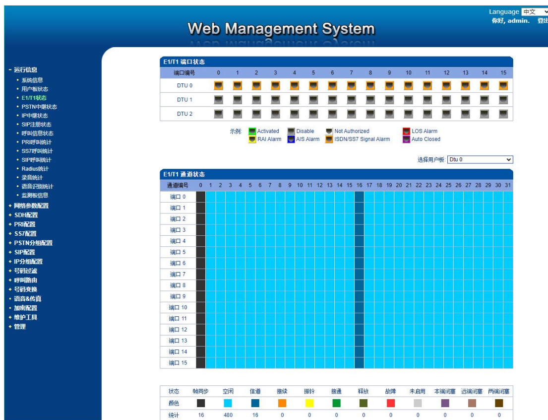
图3-3-4 E1/T1 状态
