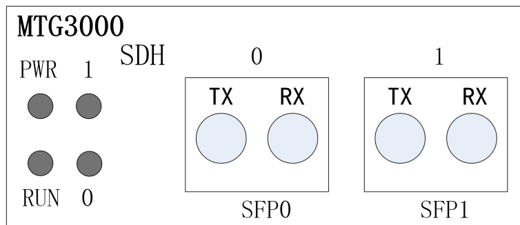
图1-2-7 SDH接口
